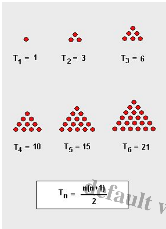
Driehoeksgetallen en de bijbehorende formule
